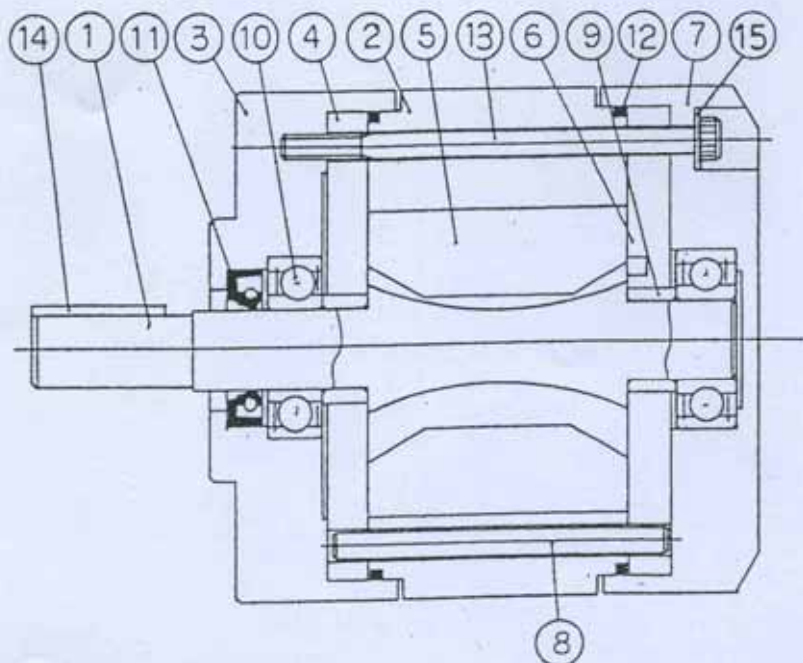
Face type
